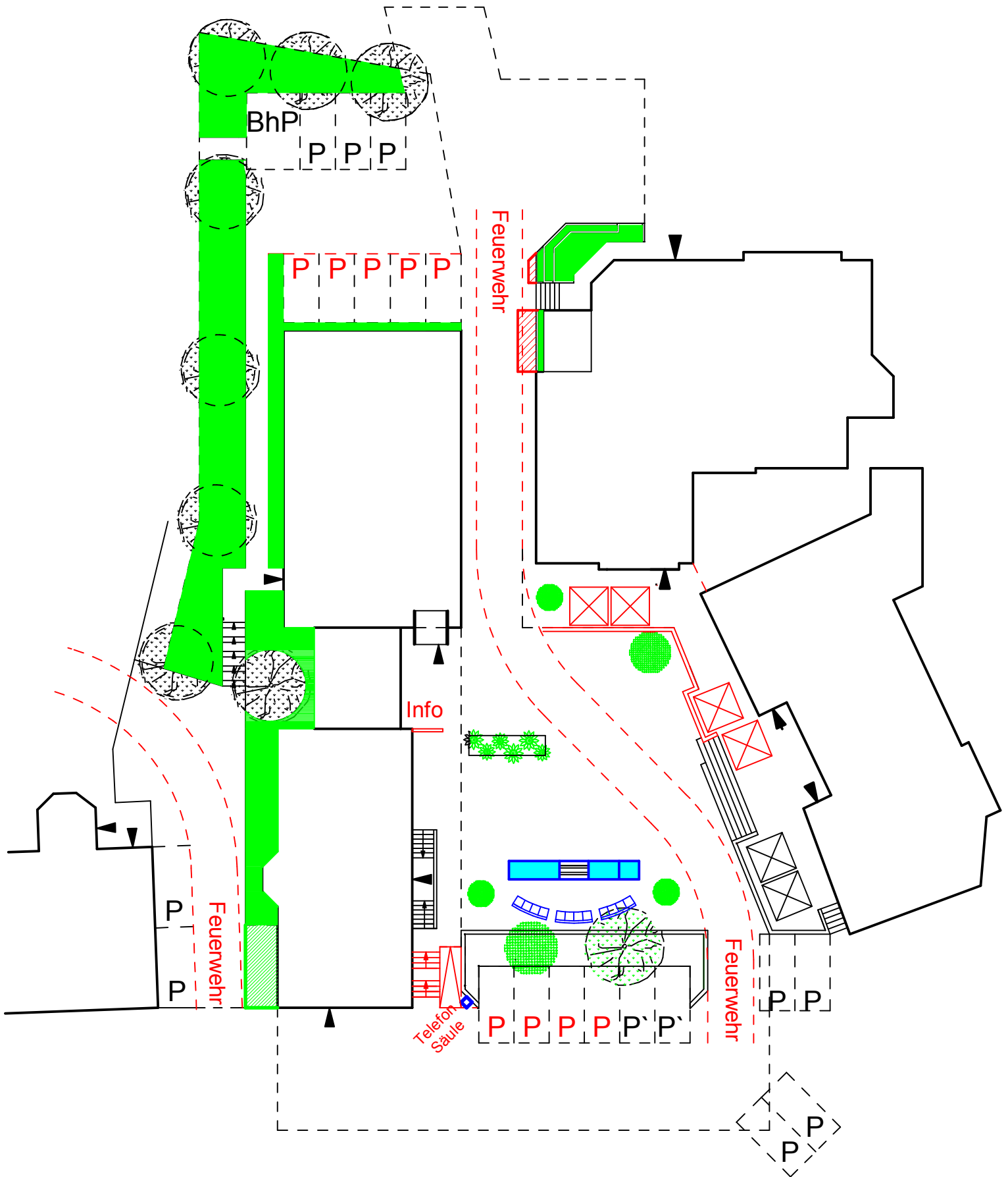
RATHAUSPLATZ Gestaltungsvorschlag P1 Treffpunkt der Bürger Visitenkarte der Gemeinde 21 Parkplätze rund um den Platz (+ 9) M = 1:325 H.Matzky Dipl.-Ing.(FH) Mai 2013
